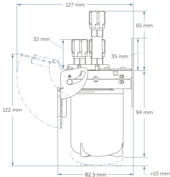
インパクト 2 V2 フィルター装着時のインパクト 2 マニホールド
