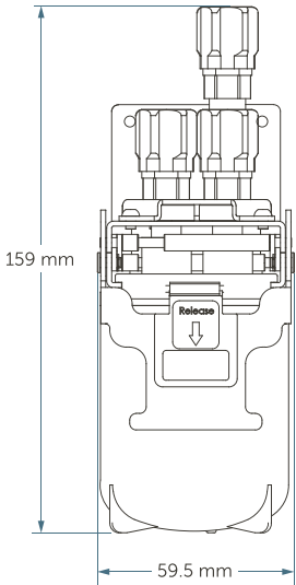
インパクト 2 V2 フィルター装着時のインパクト 2 マニホールド
