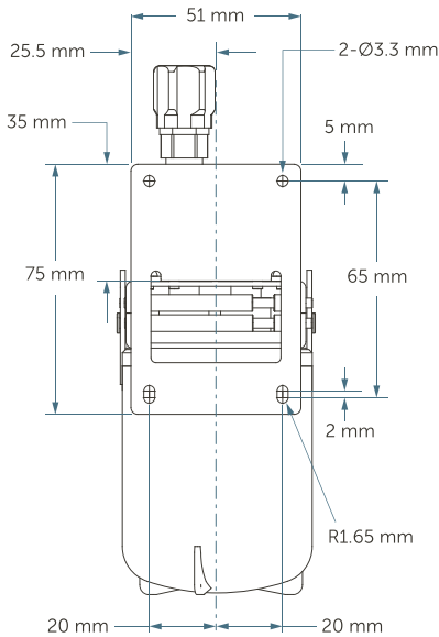
インパクト 2 V2 フィルター装着時のインパクト 2 マニホールド
