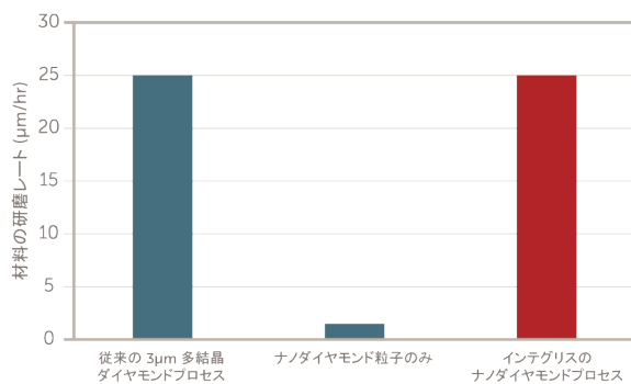
サファイアのダイヤモンドラッピングにおける研磨レート
