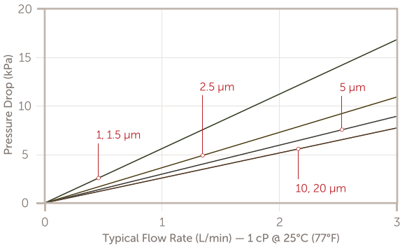
Processgard PDP Plus Mini Disposable Filters In/Out ¼ Compression Seal
