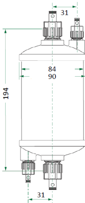
入口出口 9.53 mm (3/8") スーパー300 タイプピラー
