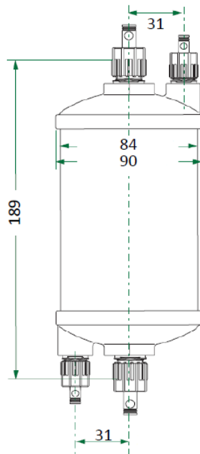
入口出口 12.7 mm (1/2") スーパータイプピラー
