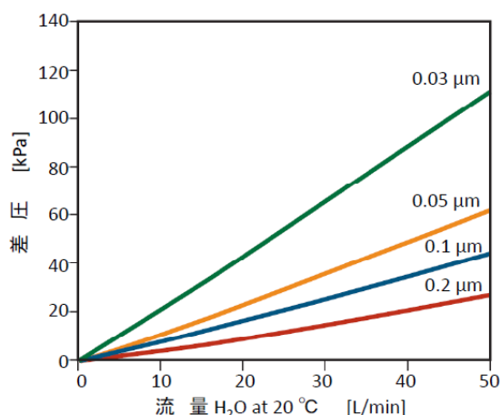
入口出口サイズ 25.4 mm (1")
