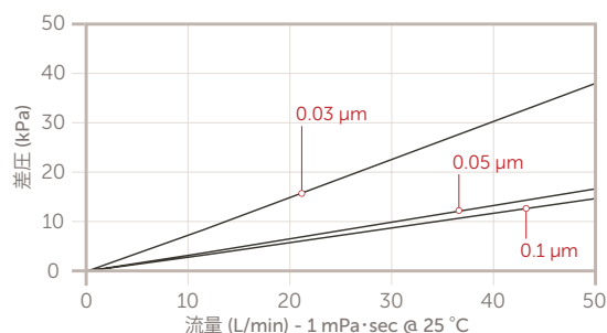
トリンジック HCE 10 インチタイプ カートリッジフィルター
