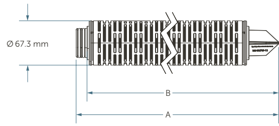
コード 5: O-リング規格 SA568-222、フィン付き
