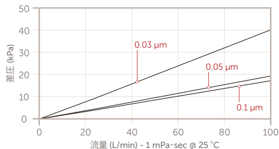
トリンジック HCE 20 インチタイプ カートリッジフィルター
