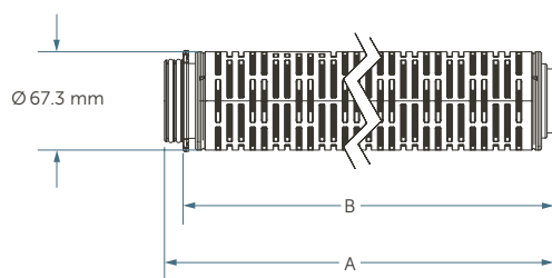
コード 6: O-リング規格 SA568-226、フラットエンド
