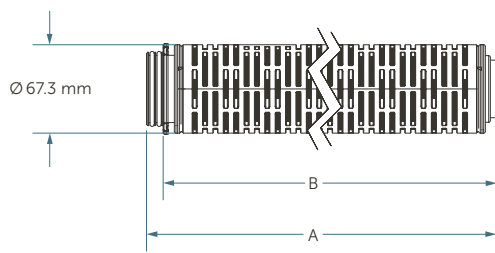
コード 6 (O-リング規格 AS568-226)
