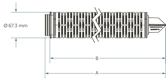
コード 7 (O-リング規格 AS568-226、フィン付き)
