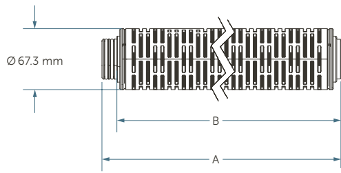
コード 0 (O-リング規格 AS568-222)
