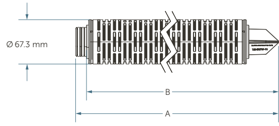
コード 5 (O-リング規格 AS568-222、フィン付き)
