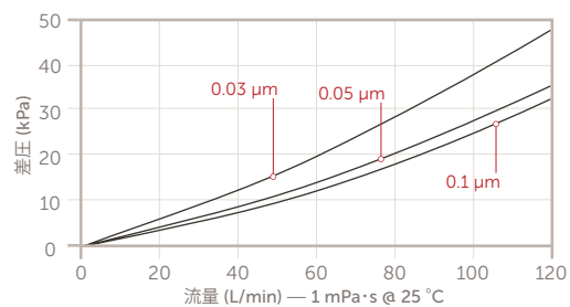
トリンジック HCM 30 インチタイプ カートリッジ
