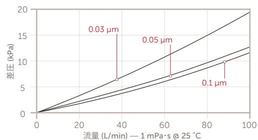
トリンジック HCM 20 インチタイプ カートリッジ
