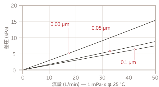
トリンジック HCM 10 インチタイプ カートリッジ
