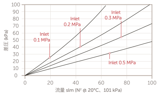
ウェハーガード III NF ミニ XL 6.35 mm ガスケット シール (1/4" VCR 互換) WG3NS2RR4
