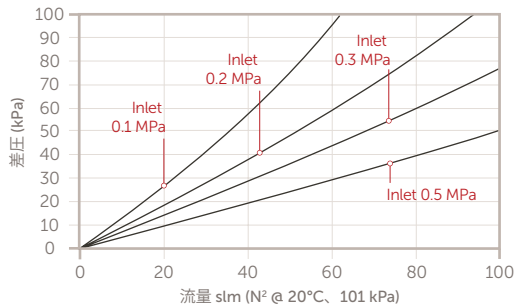
ウェハーガード III NF ミニ XL 12.7 mm ガスケット シール (1/2" VCR 互換) WG3NS2RR2
