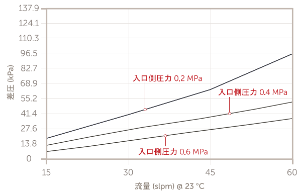
ウェハーガード IV HF ミニ ¼" (6.35 mm) ガasketシール WGL045HS3R2
