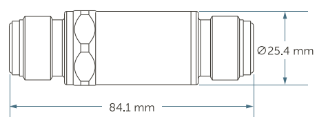
WGL045HS3R4 入口/出口 ½" (12.7 mm) ガasketシールオス
