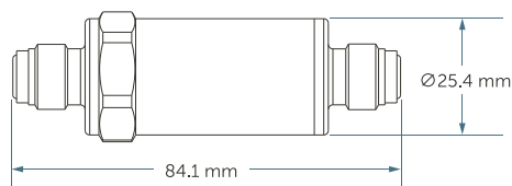
WGL045HS3R2 入口/出口 ¼" (6.35 mm) ガasketシールオス
