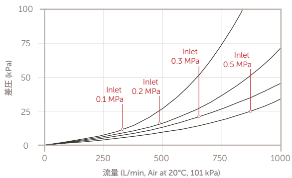
ウェハーガード MAX-1000: WGMXLBRR4, WGMXLBSS4
