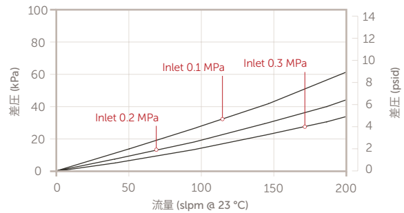
ウェハーガード SG PAL ガス フィルター YY5032PS1 9.53 mm (3/8") コンプレッションシール YY5032PR1 12.7 mm (1/2") ガasketシール
