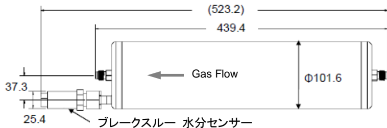
2500KH (12.7 mm ガasketシール オス (1/2" VCR 互換))
