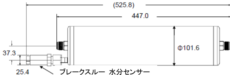
2500KH (6.35 mm ガasketシール オス (1/4" VCR 互換))
