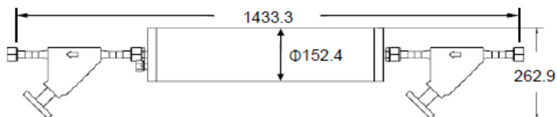
10MH (19.05 mm ガasketシール メス (3/4" VCR 互換))
