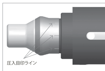
正しいインサートの取り付け方向
