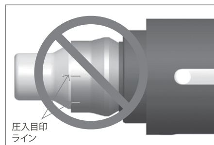
誤ったインサートの取り付け方向
