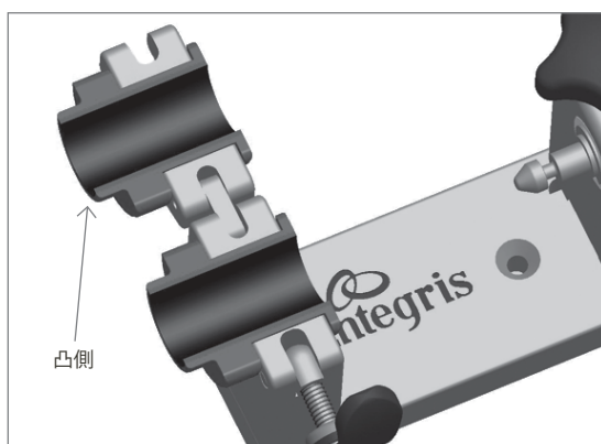
正しいゴム付きクランプインサートの取り付け方向
