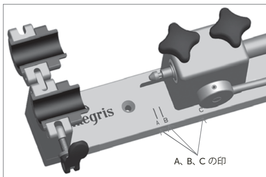
スペースが限られている場合のゴム付きクランプインサートの取り付け方向
