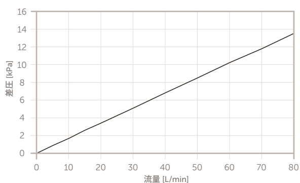
トリンジック UPW T015 40 インチタイプ カートリッジ
