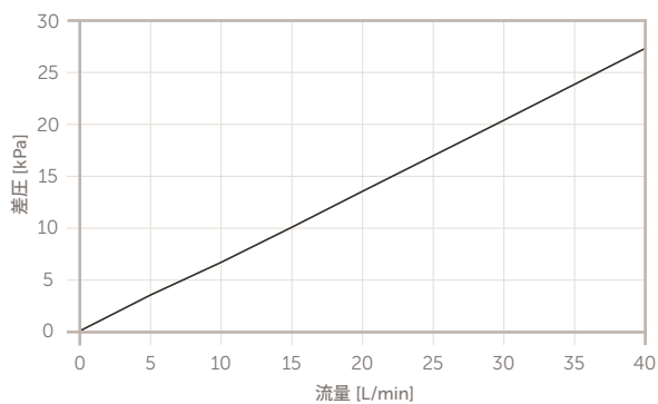
トリンジック UPW T015 10 インチタイプ カートリッジ
