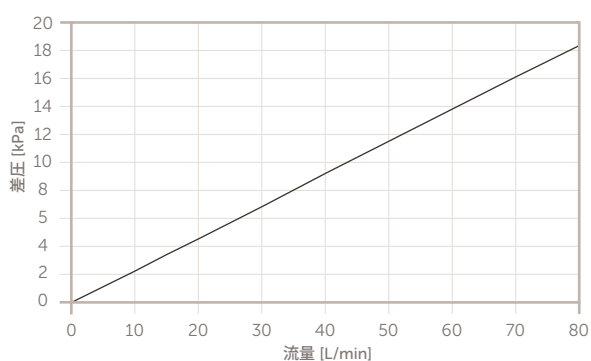
トリンジック UPW T015 30 インチタイプ カートリッジ
