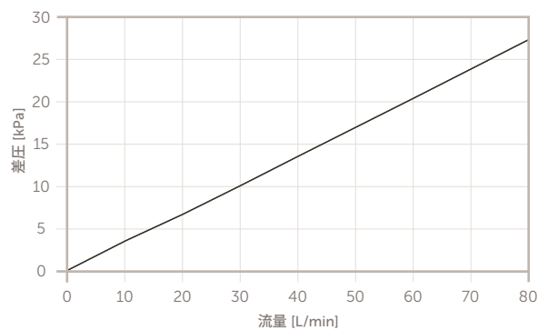
トリンジック UPW T015 20 インチタイプ カートリッジ
